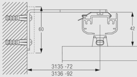
正面付 3135・3136 補助金具L型と2616ブラケット使用
