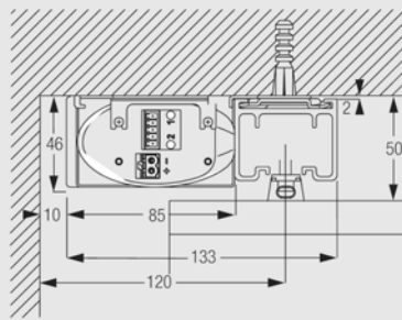
天井付 3033 クランプ使用
