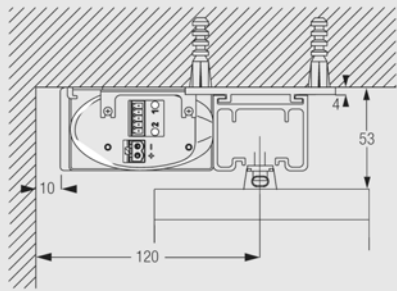
天井付 2987 ツイストブラケット使用
