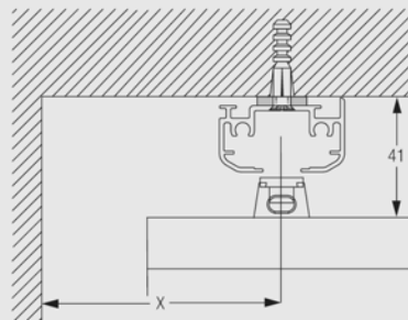
天井付 Y0414 座金使用
