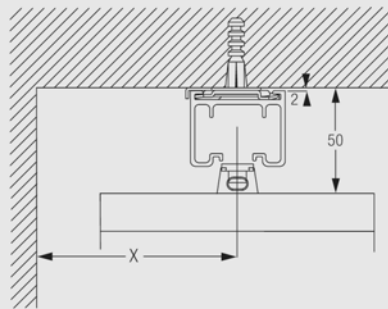
天井付 3033 クランプ使用
