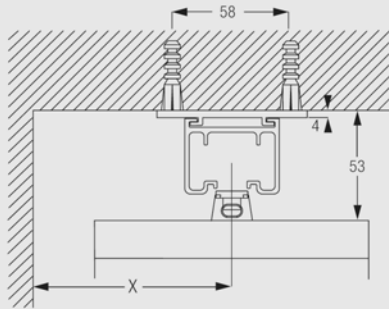
天井付 2987 ツイストブラケット使用
