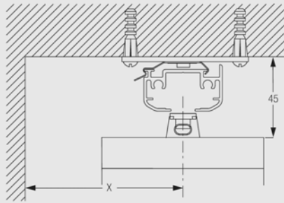
正面付 3135・3136 補助金具L型と2616ブラケット使用
